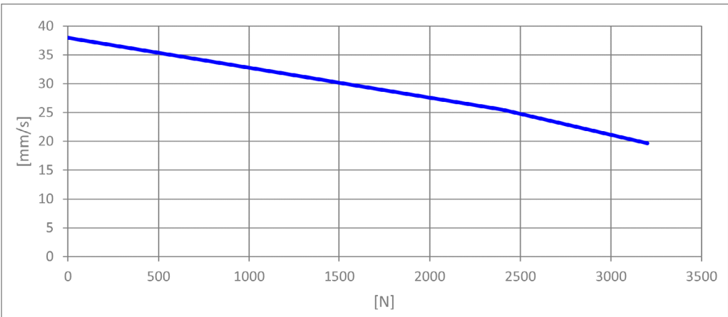
图3 搭载CBD6S的四升降柱（均摊负载） — 300W
