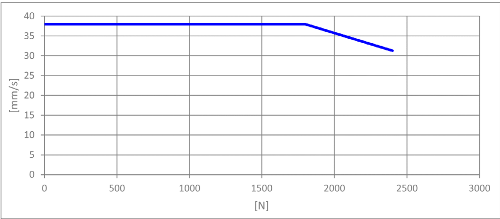
图2 搭载CBD6S的三升降柱（均摊负载） — 300W
