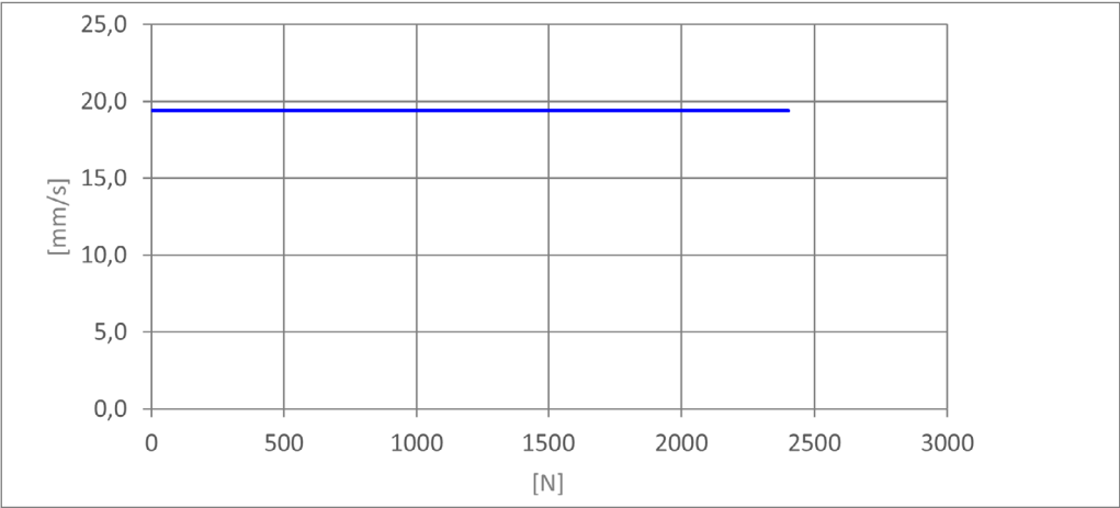
图4 搭载CBD6S的双升降柱（均摊负载）— 200W/300W
