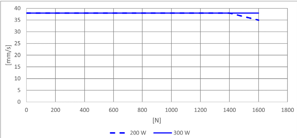
图1 搭载CBD6S的双升降柱（均摊负载） — 200W/300W
