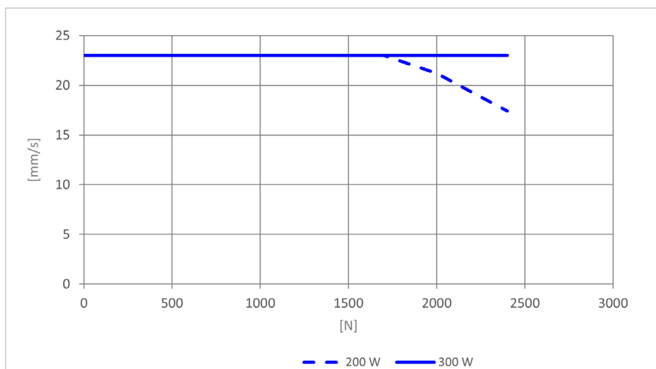
图7 搭载CBD6S (200W/300W) 的2根DL6升降柱(均衡负载)的性能曲线图
