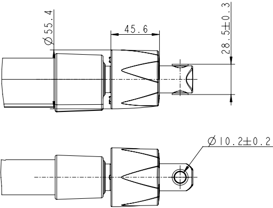
头部连接件 (选项: P, 带衬套)
