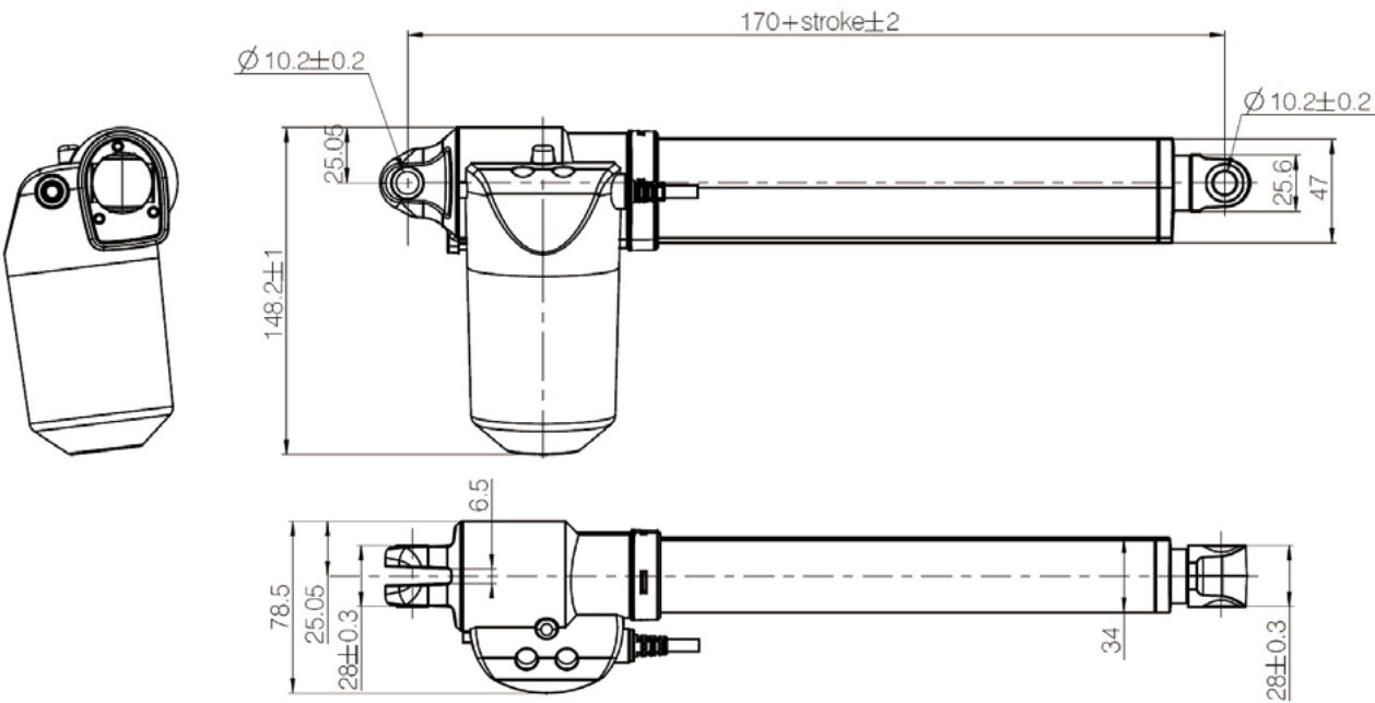
KA30（带有旋转90° 的背部连接件的标准电机）
