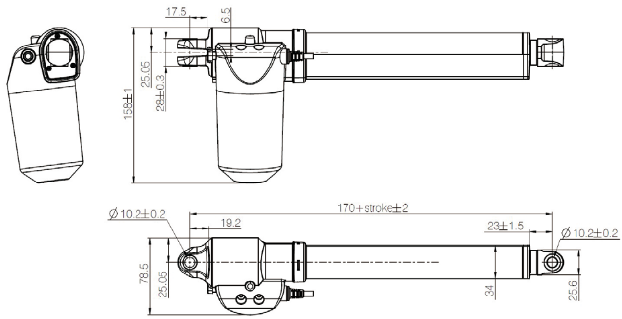
KA30（带有标准背部连接件的大型电机）
