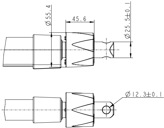
头部连接件 (选项: P, 不带衬套)
