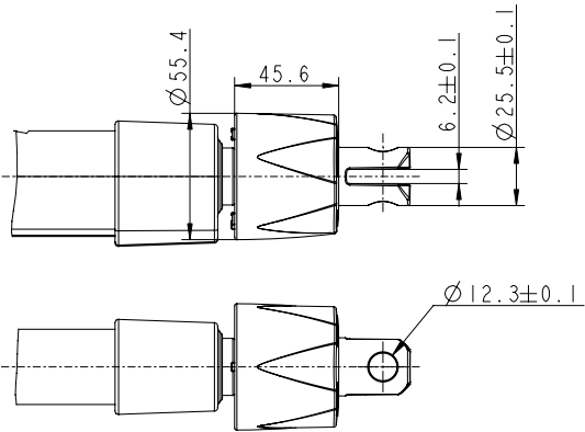
头部连接件 (选项: Q, 不带衬套)
