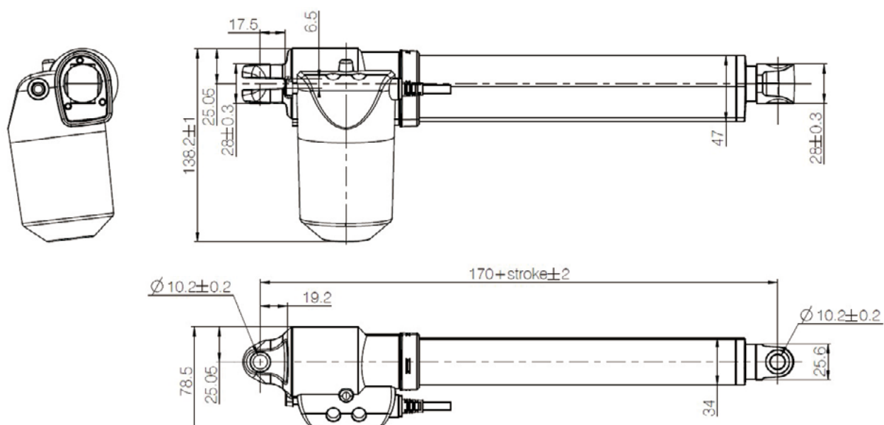
KA30 (带有标准背部连接件的小型电机)
