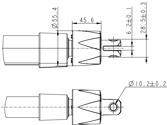
头部连接件 (选项: Q, 带衬套)
