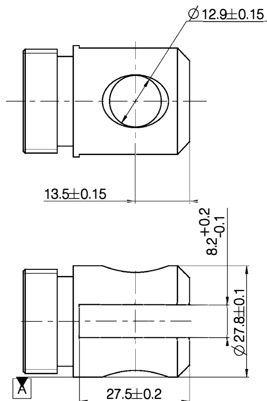
力纳克 P/N: 0361275 AISI 304
