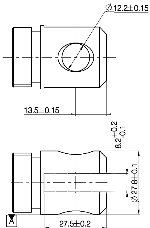
力纳克 P/N: 0361260 AISI 304
