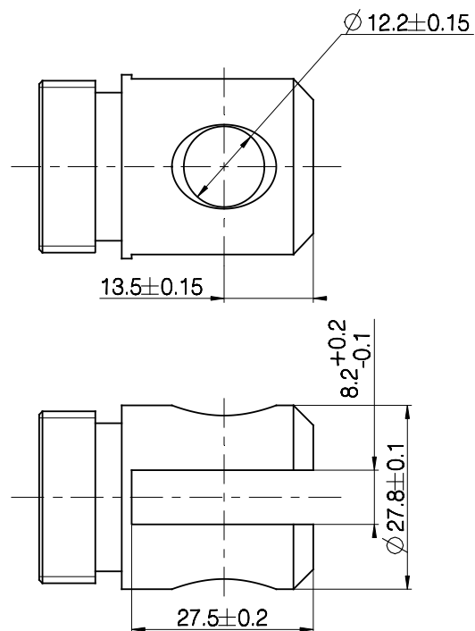
力纳克 P/N: 0361138 易切削钢镀锌表面
